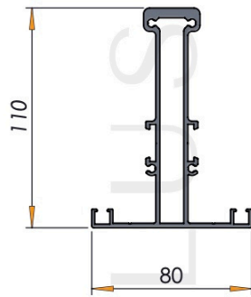
KROKIEW ZX005
