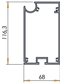
BELKA ZX004
