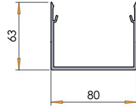
SŁUP 63 ZX003
