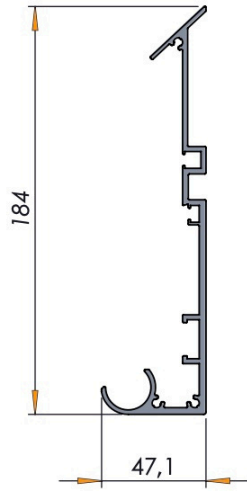
NAŚCIENNY ZX001
