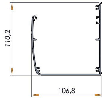
RYNNA ZX006
