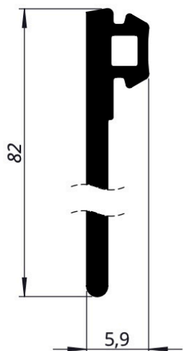
USZCZELKA U003
