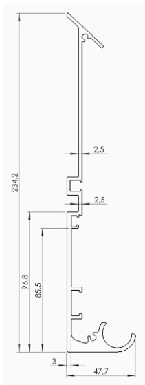
NAŚCIENNY PR001
