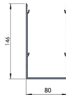
SŁUP 146 ZX002
